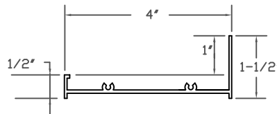
FLANGE FRAME JAMB
